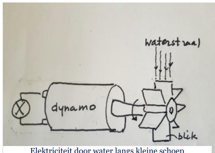
Elektriciteit door water langs kleine schoep
